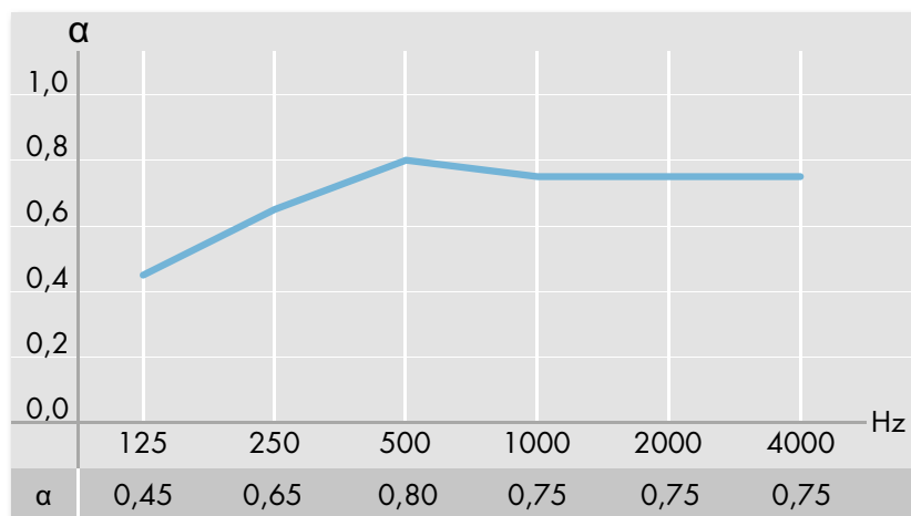
Plénum 200 mm, sans laine minérale (CSTB)
